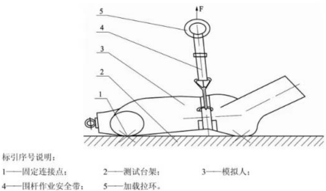
图 C.3 围杆作业安全带整体静负荷试验示意图
