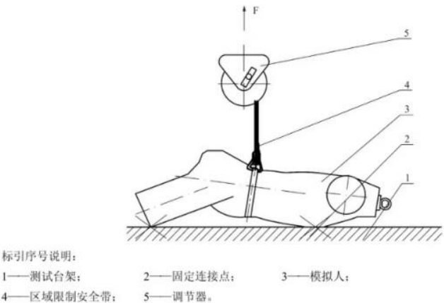
图 C.1 安全带静负荷试验示意图
